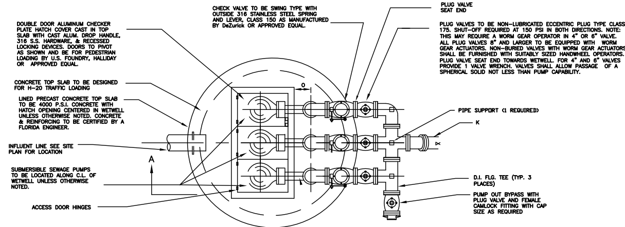
WETWELL - PLAN N.T.S.
