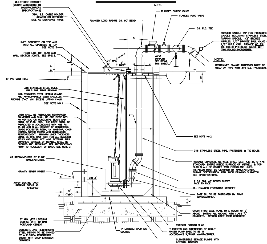
WETWELL - ELEVATION SECTION A-A N.T.S.
